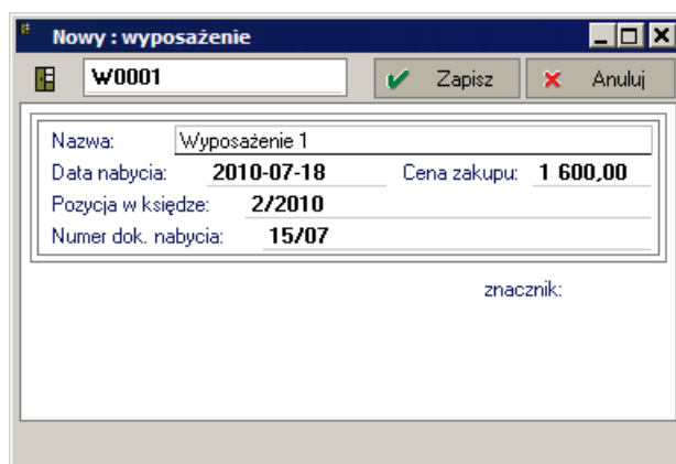
Rys. 5-26 Okno Wyposażenie.
