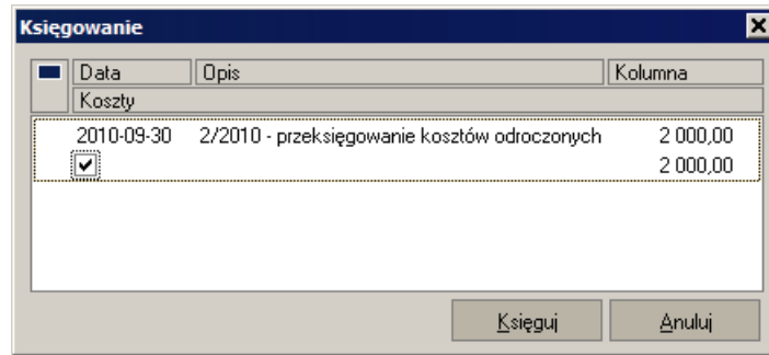
Rys. 7-11 Dialog Księgowanie .
