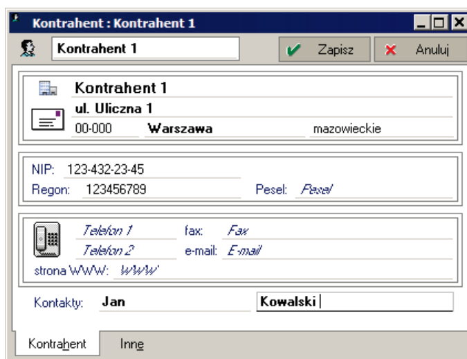
Rys. 5-6 Okno Kontrahent.
